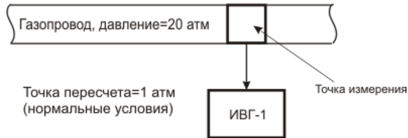
Рисунок 5.4 Пример использования пересчета показаний влажности.
