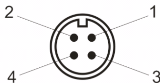
Рисунок 3.2 Разъем подключения преобразователей влажности
